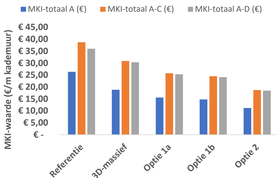
Figuur 3. MKI-reductie van (deels) Computational Design ontworpen kademuur-elementen.
