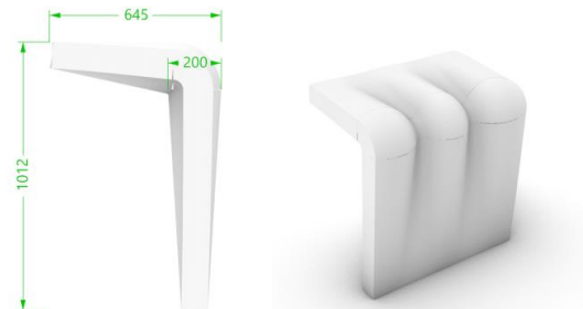
Figuur 7: Ontwerp optie 2 (printbreedte: 100 mm).
