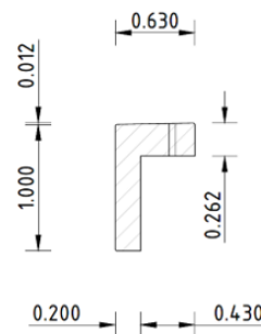
Figuur 1: Afmetingen referentie-element.
