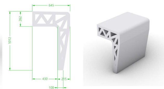
Figuur 5: Ontwerp optie 1b (printbreedte: 50 mm).
