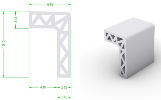
Figuur 4: Ontwerp optie 1a (printbreedte: 50 mm).
